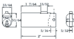
5002LP
