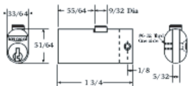
5001LP
