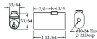
EXP-19DC
